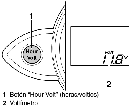
SJU37271 Indicador de nivel de combustible
