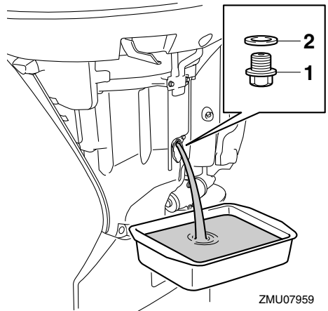
1. Parafuso de escoamento 2. Junta
