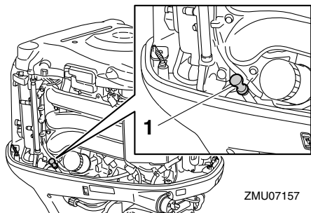
1. Öljymäärän mittatikku
