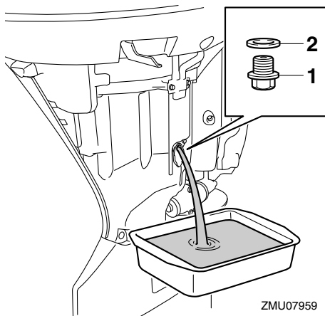
1. Aftapschroef 2. Pakking
