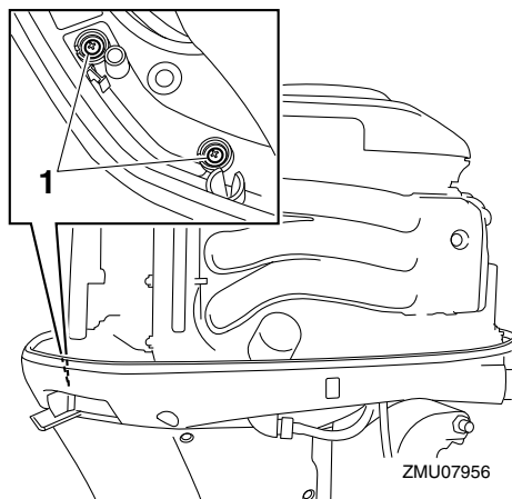
1. Schroef
