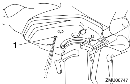
1. Kühlwasser-Kontrollstrahl
