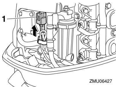
1. Wasseranzeigeschalter-Stecker
