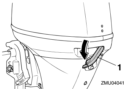
1. Haubenverriegelungshebel
