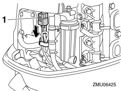
1. Wasseranzeigeschalter-Stecker
