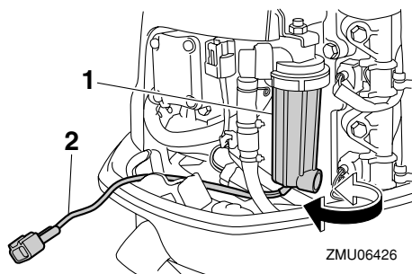
1. Halter
