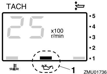
1. Öldruck-Warnanzeige
