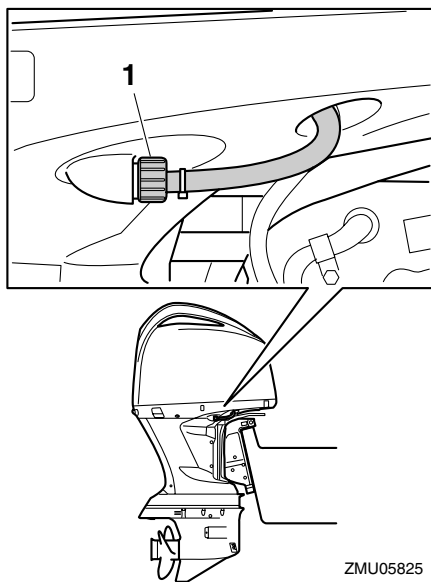
1. Doorspoelplug
