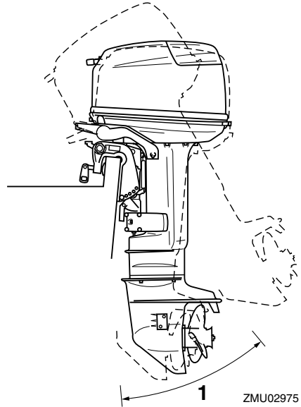
1. Trimm-Betriebswinkel
