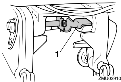
1. Kipperrhebel
