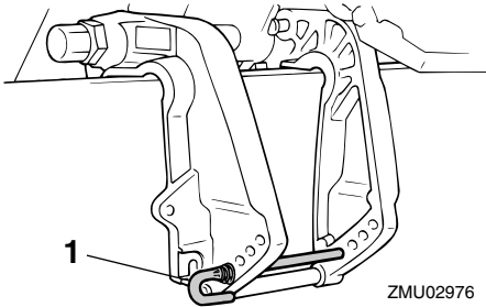
1. Trimmstange
