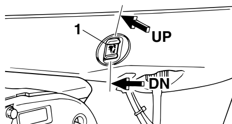
1. Interruptor de elevación y trimado del motor
