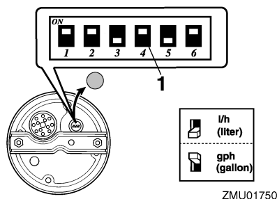
1. Interrupteur de programmation
