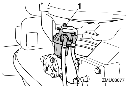
1. Mutteri
