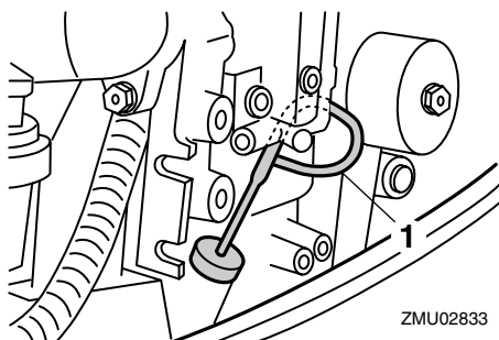
1. Oljemätsticka
