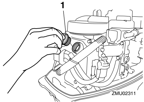
1. Oljepåfyllningskåpa
