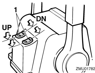
1. Interruttore PTT
