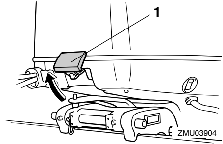
1. Motorkapvergrendelingshendel(s)
