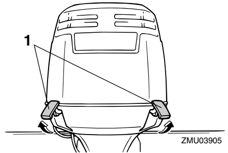
1. Motorkapvergrendelingshendel(s)
