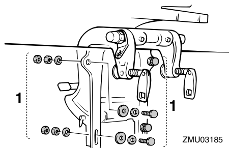
1. Boulons
