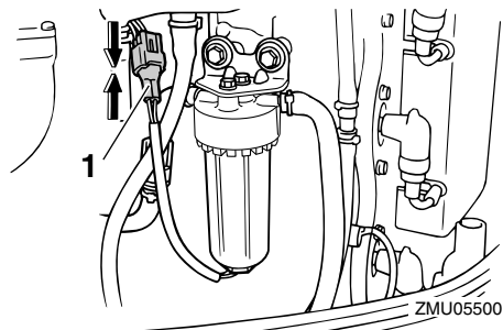
1. Coupleur du capteur de présence d'eau
