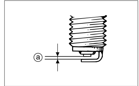
a. Folga da vela de ignição
