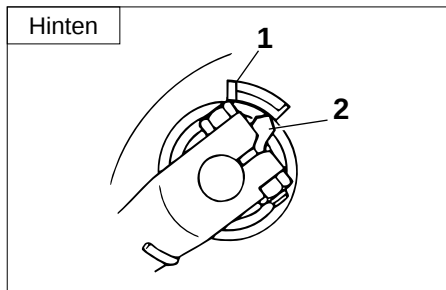
1. Verschleißgrenze 2. Trommelbremsbeläg-Verschleißanzeiger
