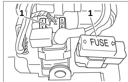
1. Sicherungskasten (x2)
