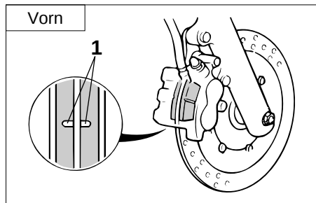
1. Scheibenbremsbeläg-Verschleißanzeiger
