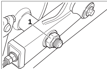
1. Achsmutter
