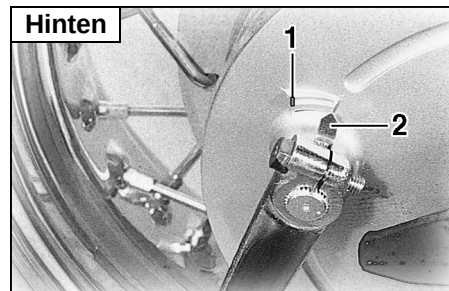
1. Verschleißgrenze 2. Trommelbremsbelag-Verschleißanzeiger
