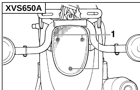
1. Schraube (× 3)
