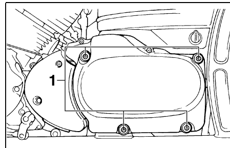
1. Schraube (× 4)
