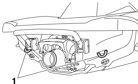
1 Δακτύλιος πρύμνης
