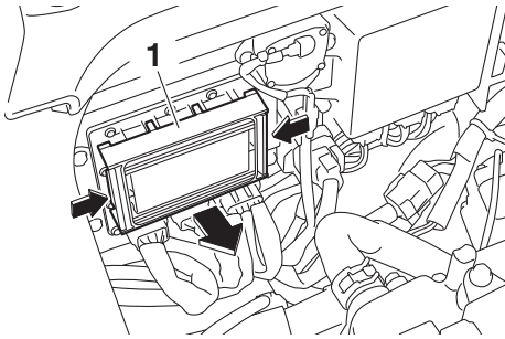
1 Καπάκι ασφαλειοθήκης
