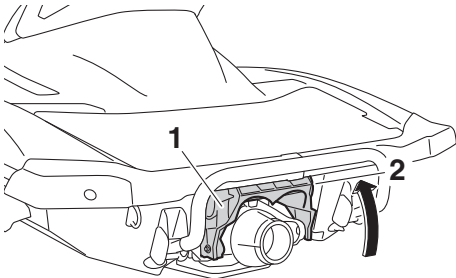
1 Τύμπανο αναστροφής (όπισθεν) 2 Θέση εμπροσθοπορείας
