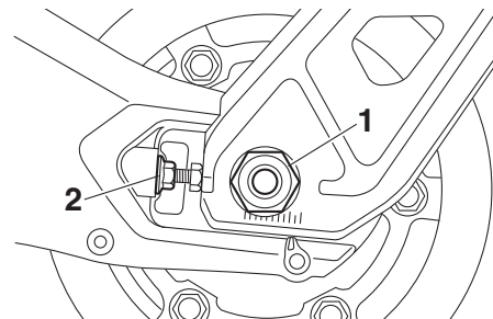
1. Wielascoer
