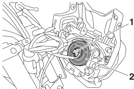
1. Accoppiatore del faro 2. Coprilampada del faro
