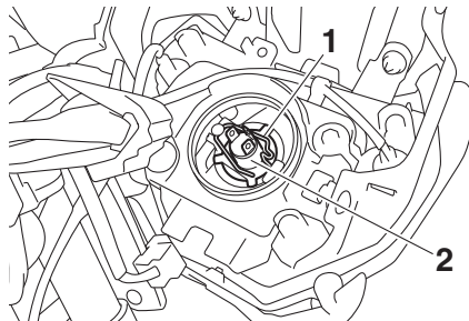
1. Portalampada del faro 2. Lampadina del faro
