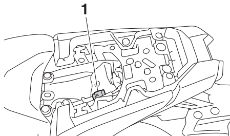
1. Connettore diagnostica
