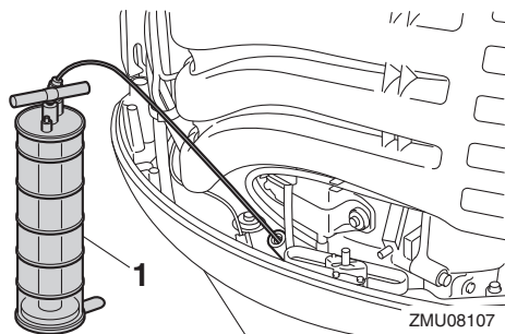
1. Cambiador de óleo
