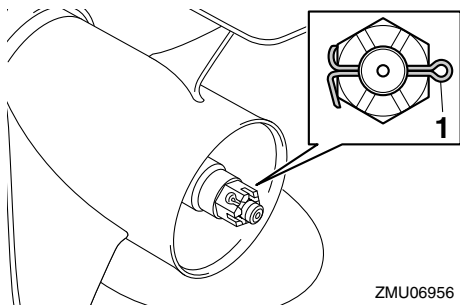
1. Sokka
