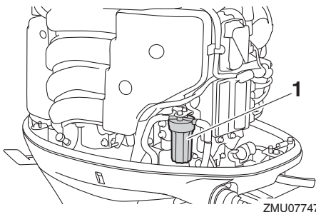
1. Brandstoffilter
