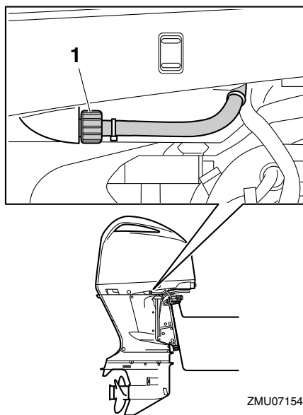
1. Spülanschluss
