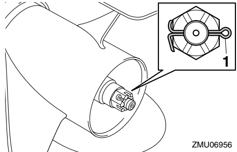
1. Sicherungssplint
