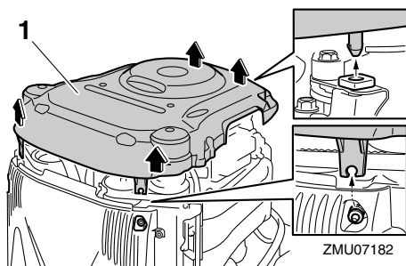
1. Coperchio del magnete volante
