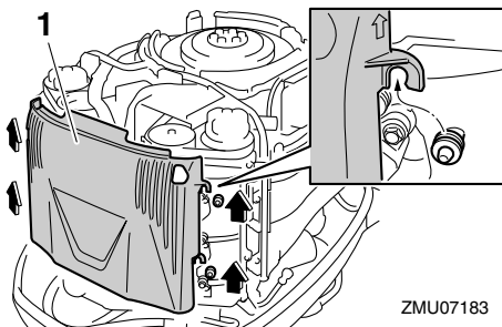
1. Coperchio del modulo ECM (modulo di comando elettronico)
