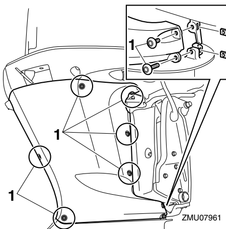
1. Schraube
