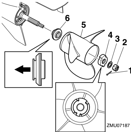
1. Sicherungssplint
