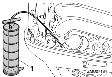
1. Ölwechsler
