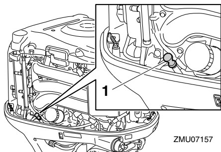
1. Ölmesstab
