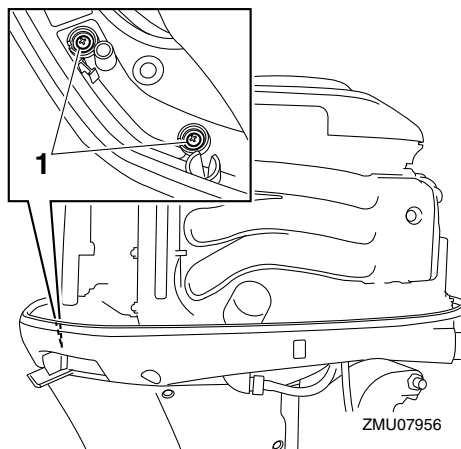
1. Schraube
