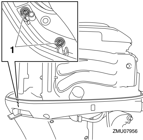
1. Schraube
