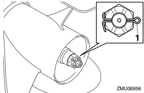
1. Sicherungssplint
