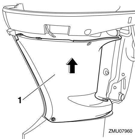
1. Schutzabdeckung
