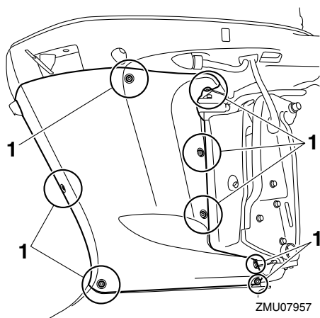
1. Schraube
