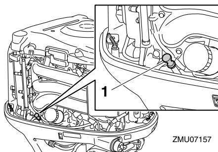
1. Oliepeilstok
