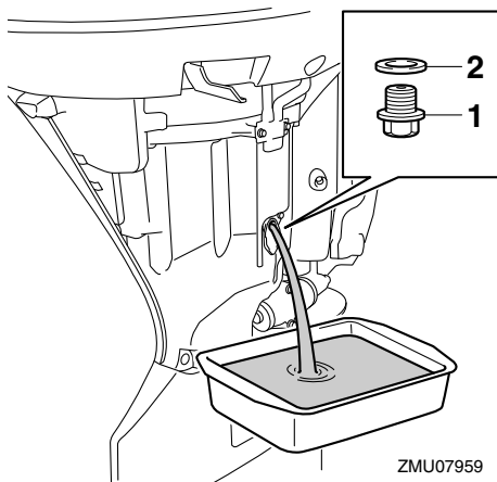
1. Aftapschroef 2. Pakking
