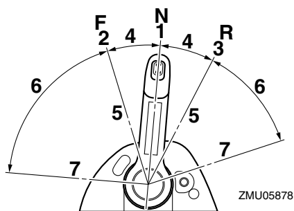
1. Neutraal “N” 2. Vooruit “F”
