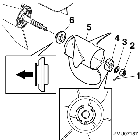
1. Splitpen
