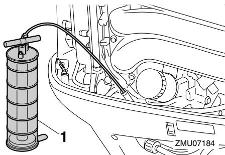
1. Olieverser
