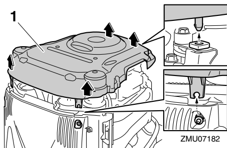
1. Vliegwielmagneetdeksel
