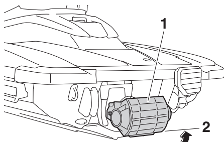
1 Inverseur
